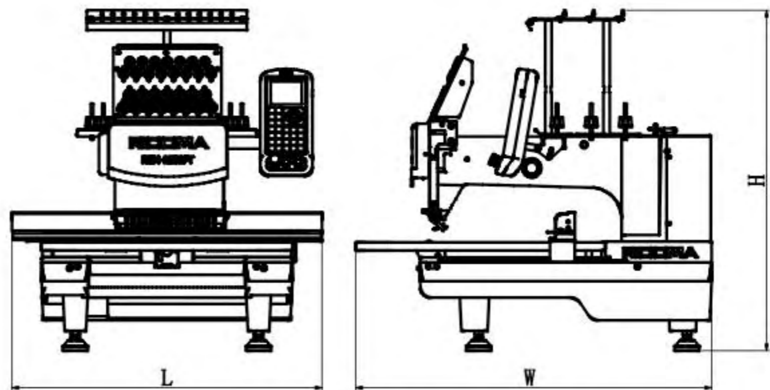
RCM-1501PT L:744 W:856 H:820 (mm)
