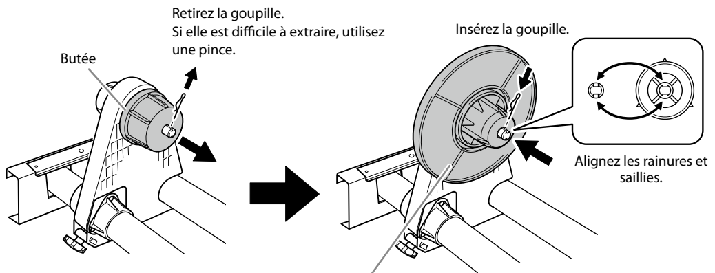
Flasque pour rouleaux avec un tube de 2" de diamètre
