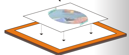
Placer une feuille de protection sur le plateau inférieur de la presse pour éviter de le marquer
